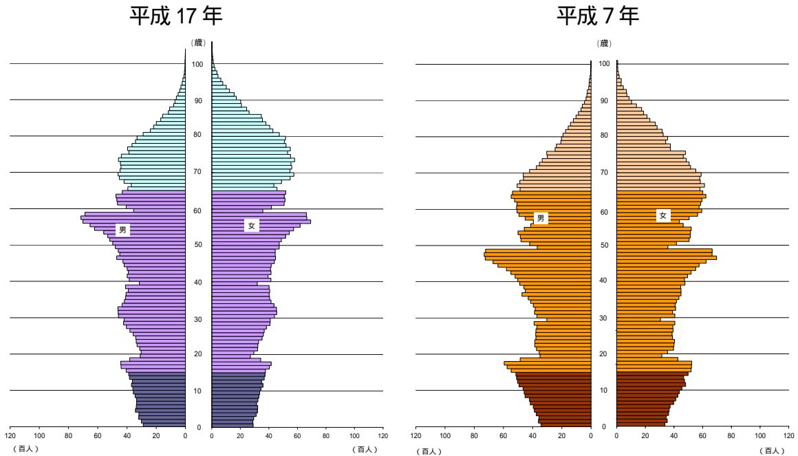
図2 島根県の年齢（各歳），男女別人口（平成7年・17年）
