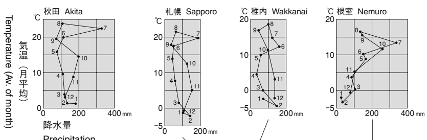
図 1-1 気温と降水量 (平成21年) TEMPERATURE AND PRECIPITATION (2009)
