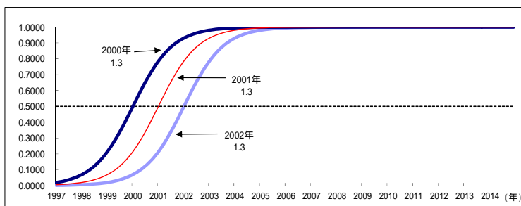
月末の曜日の重み付けに使用したロジスティック曲線の概形
