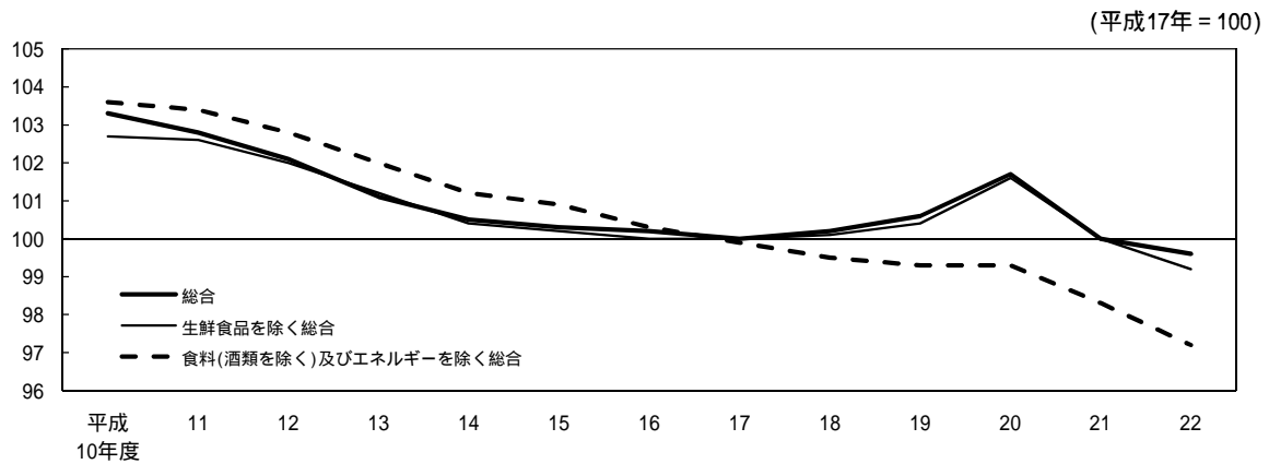
図10 指数の動き
